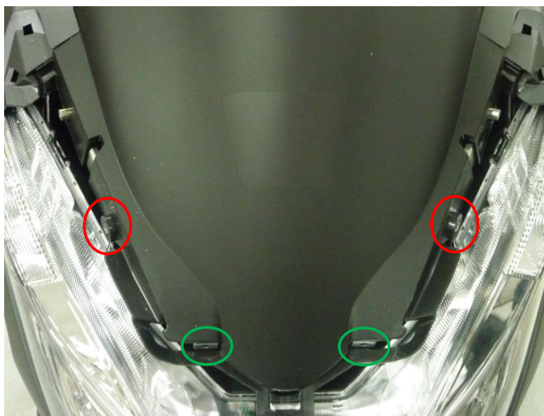
Position des vis de fixation du cache d'origine en vert Position des entretoises plastique en rouge
