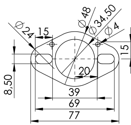
S.s. flange Cod.206443
