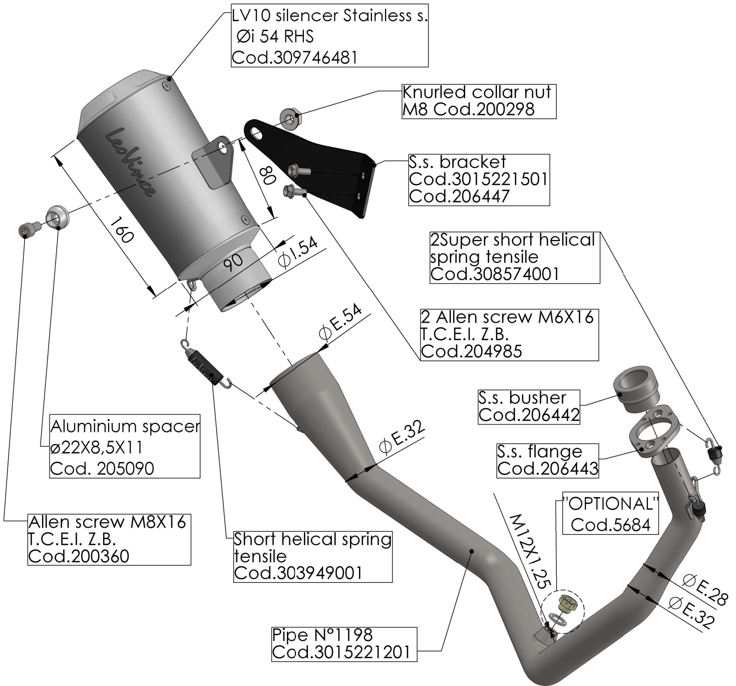
S.s. flange Cod.206443
