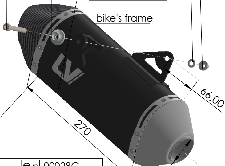
S.S. Muffler P/N 3015601485
